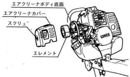
エアクリーナボディ底面
